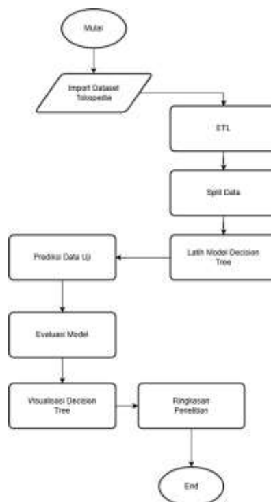
Gambar 1 Alur Metodologi
