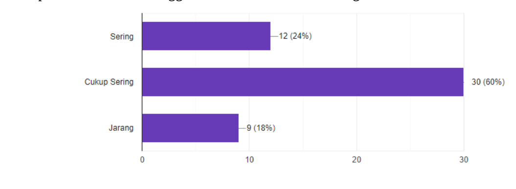
Gambar 1 : Diagram Batang Instrumen Pertanyaan “Apakah anda selalu menggunakan Bahasa Indonesia dengan baik dan benar?”
