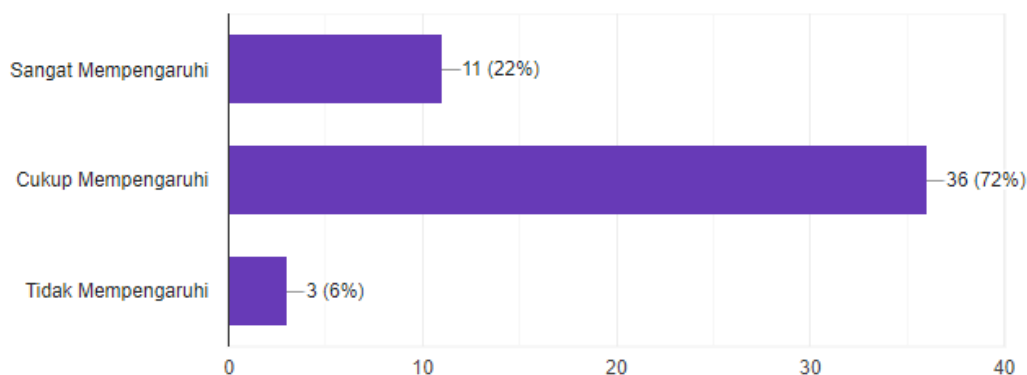
Gambar 4 : Seberapa besar pengaruh globalisasi terhadap cara anda dalam menggunakan Bahasa Indonesia?
