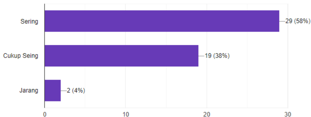
Gambar 2 :Seberapa sering anda menggunakan Bahasa Indonesia dalam kegiatan akademik?
