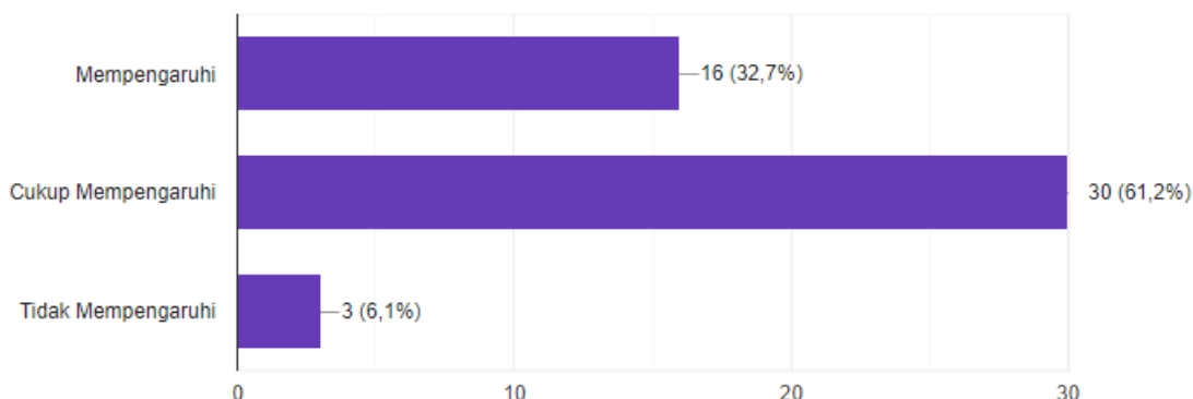
Gambar 3 :Apakah globalisasi mempengaruhi cara anda dalam menggunakan Bahasa Indonesia?
