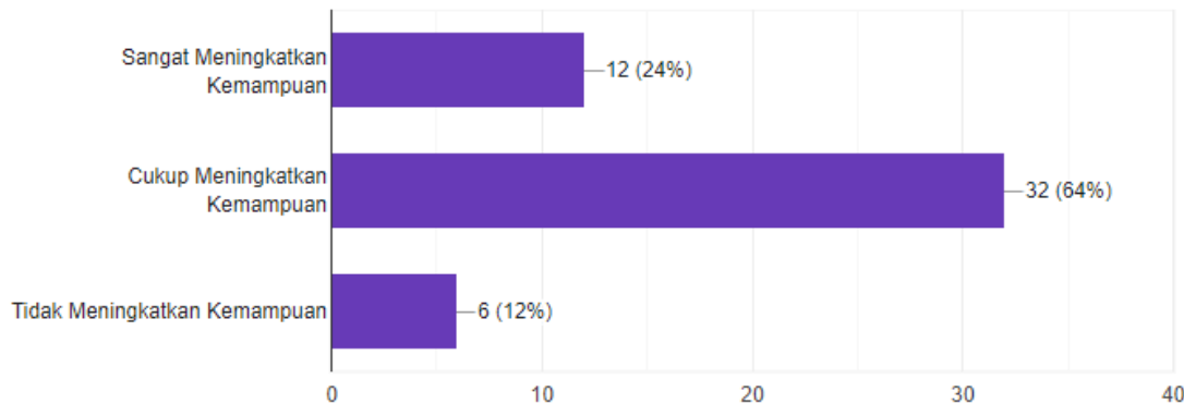
Gambar 5 :Apakah sistem akademik di Fakultas Ekonomi UNIMED mendorong meningkatkan kemampuan Bahasa Indonesia?
